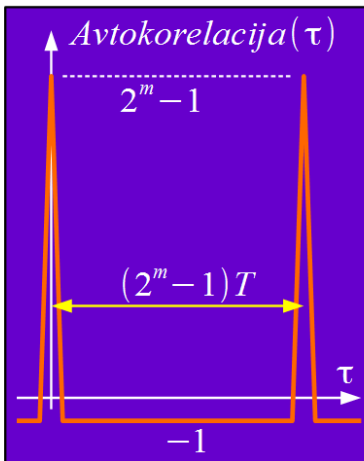
Pseudonaključna zaporedja LFSR
