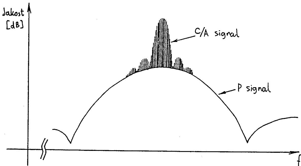
Slika 3 - Frekvenčni spekter C/A + P oddaje.
