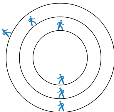
Slika 4.12: Podobnost med tekači po krožnici in kroženjem snovi znotraj galaksij[33]
