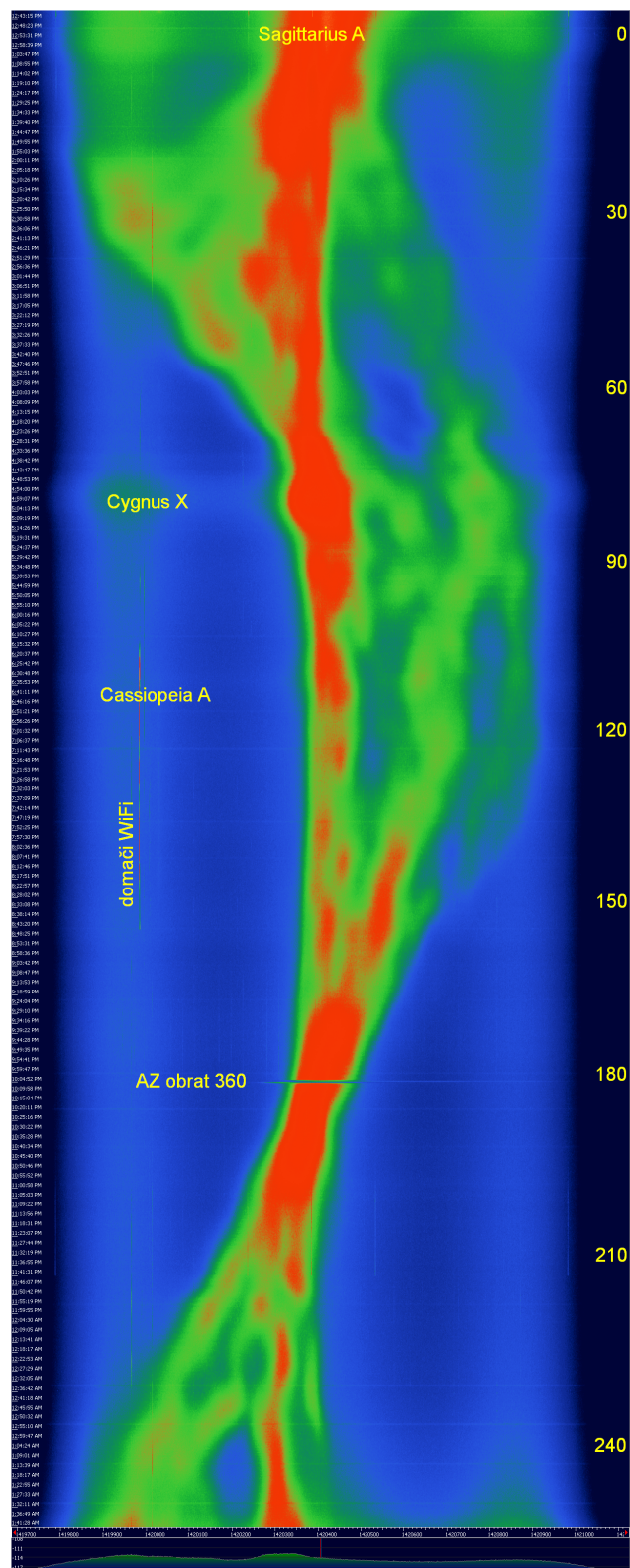
Slika 4.8: Spektar vodikove črte v galaktični ravnini
