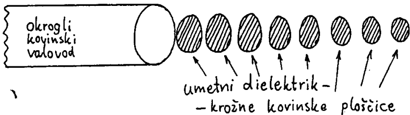
(B) Valvodni lijak z lečo iz umetnega dielektrika
