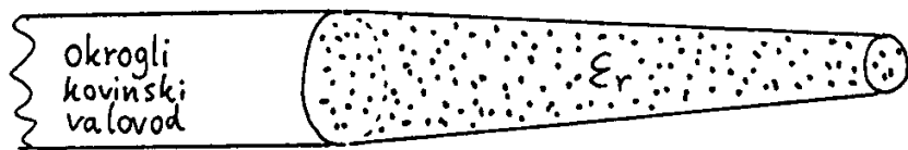
(A) Valvodni lijak z dielektrično lečo
