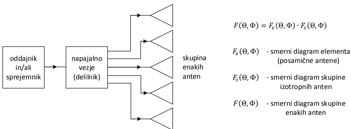
Slika 1: Skupina enakih anten
