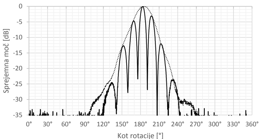
Slika 4: Smerni diagram skupine dveh anten razmaknjenih za 3\lambda .
