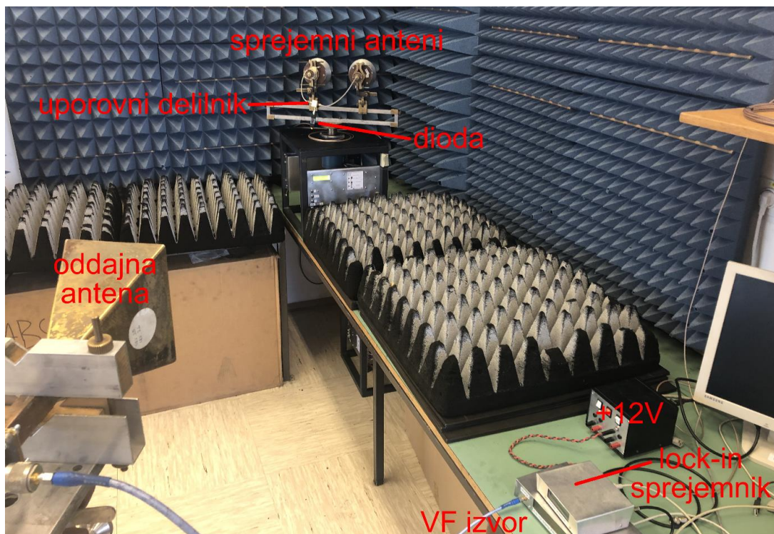
Slika 3: Slika vezave merilnih pripomočkov
