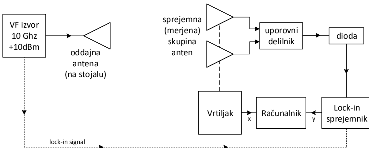
Slika 2: Skica vezave merilnih pripomočkov
