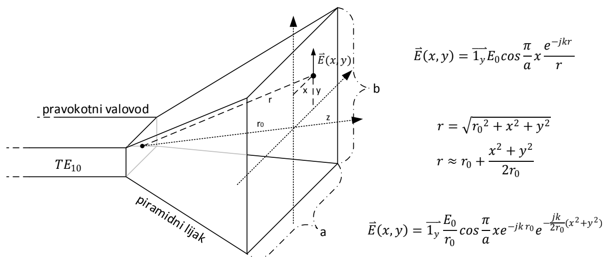
Slika 1: Porazdelitev polja na odprtini piramidnega lijaka
