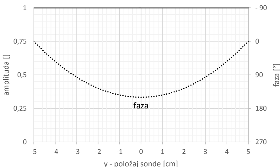
Slika 4: Porazdelitev polja na odprtini piramidnega lijaka v \vec{E} ravnini.
