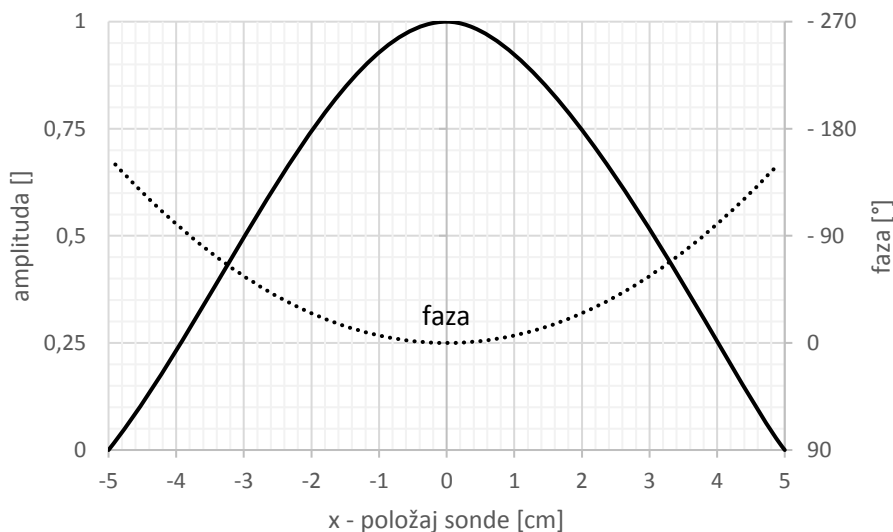
Slika 5: Porazdelitev polja na odprtini piramidnega lijaka v \vec{H} ravnini.
