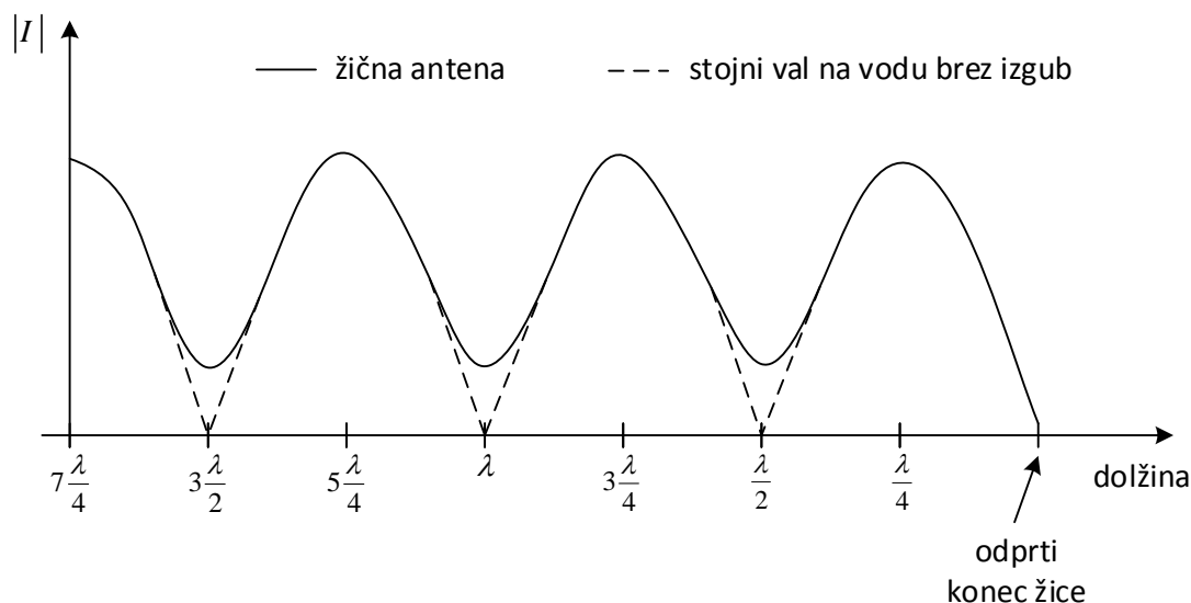
Slika 1: Porazdelitev amplitude toka na žični anteni
