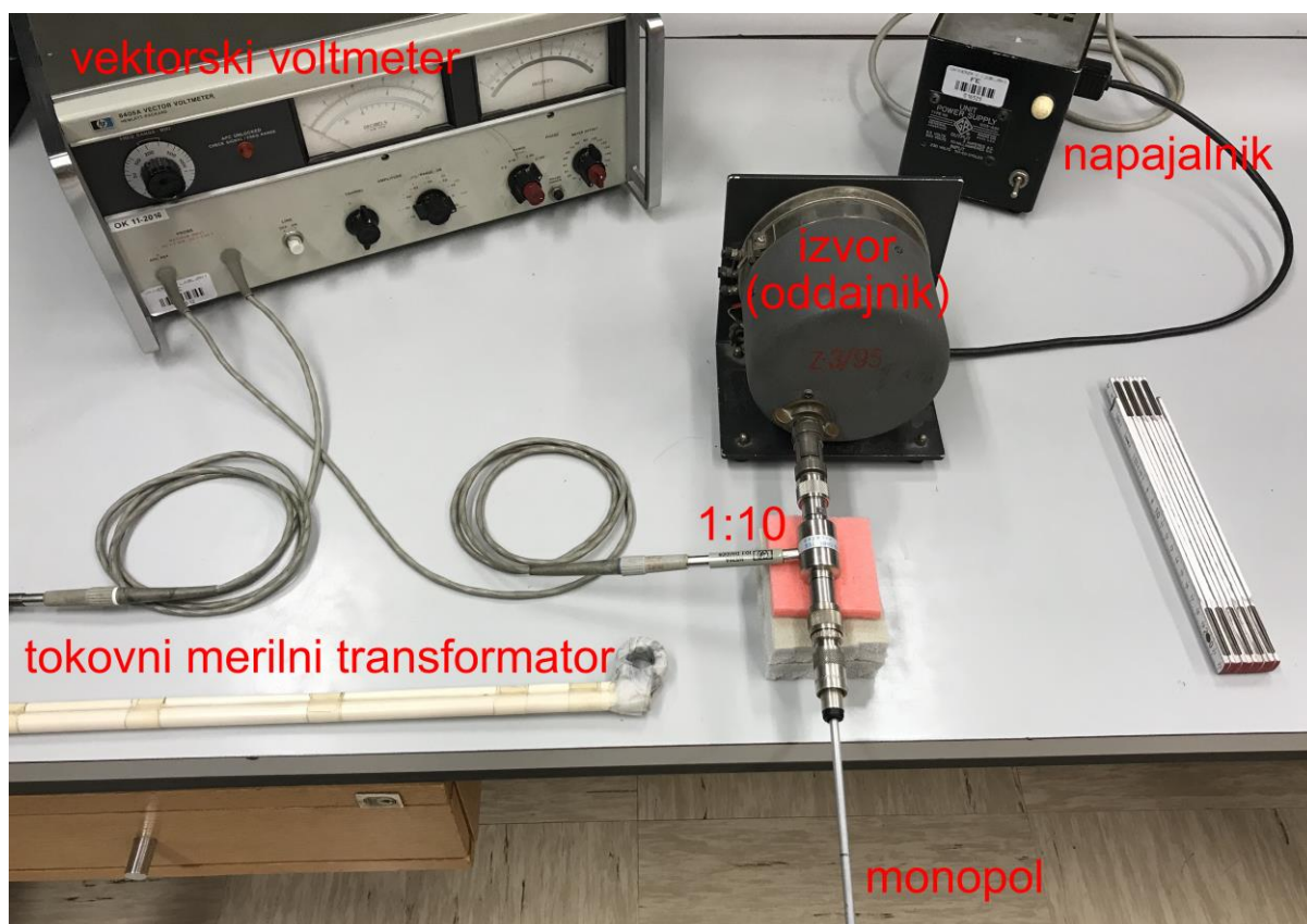
Slika 4: Slika vezave merilnih pripomočkov
