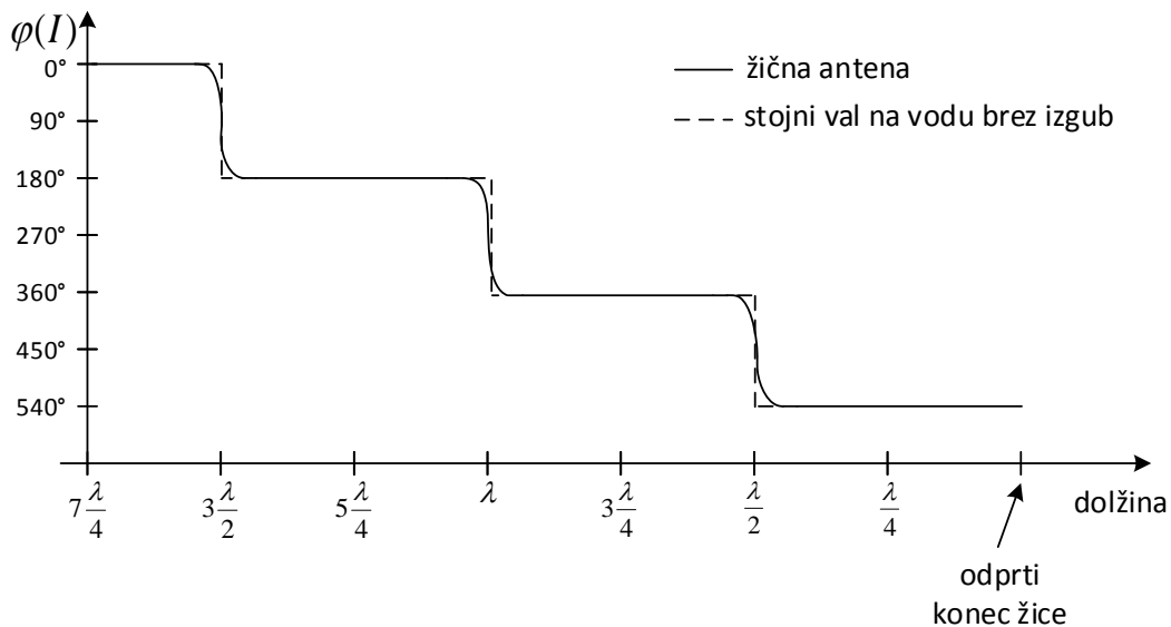
Slika 2: Porazdelitev faze toka na žični anteni
