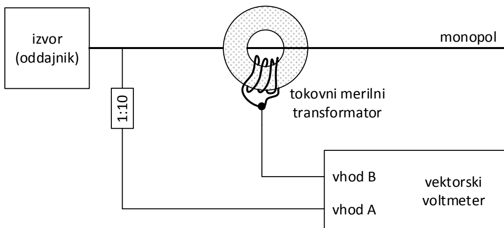
Slika 3: Skica vezave merilnih pripomočkov
