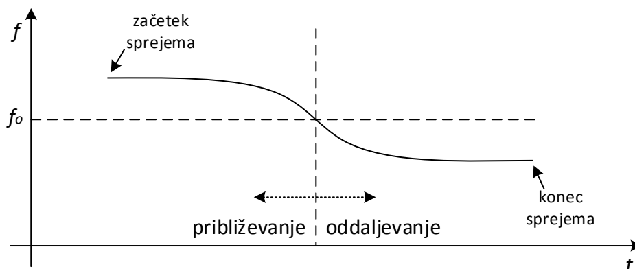
Slika 2: Časovni potek Dopplerjevega pomika pri sprejemu satelita v nizki tirnici.
